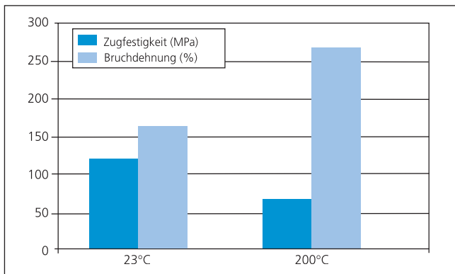
Abbildung 1: Physikalische Eigenschaften bei 23 °C und 200 °C für APTIV™ 1000, 50 µm (ISO 527)
